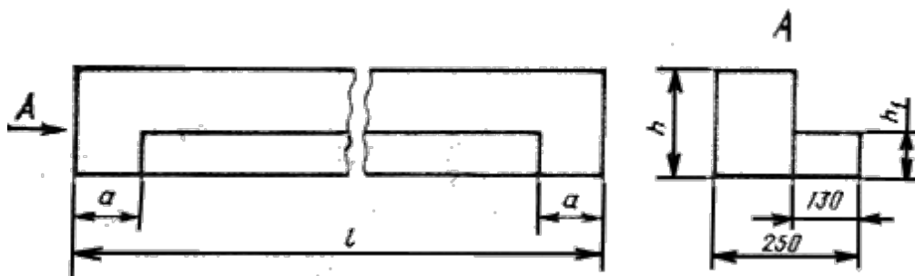
Перемычка типа ПФ
