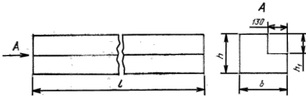
Перемычка типа ПГ
